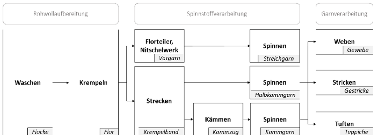
Abbildung 16: Übersicht Spinnverfahren
